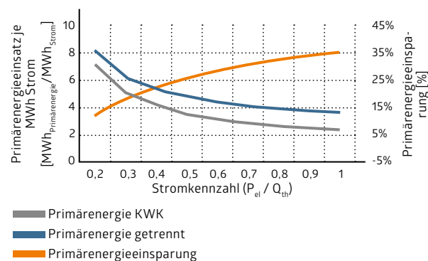
Abb. 5: KWK: Primärenergieeinsatz im Vergleich; eigene Darstellung auf Basis von Gesellschaft Energietechnik 2003: S. 101
